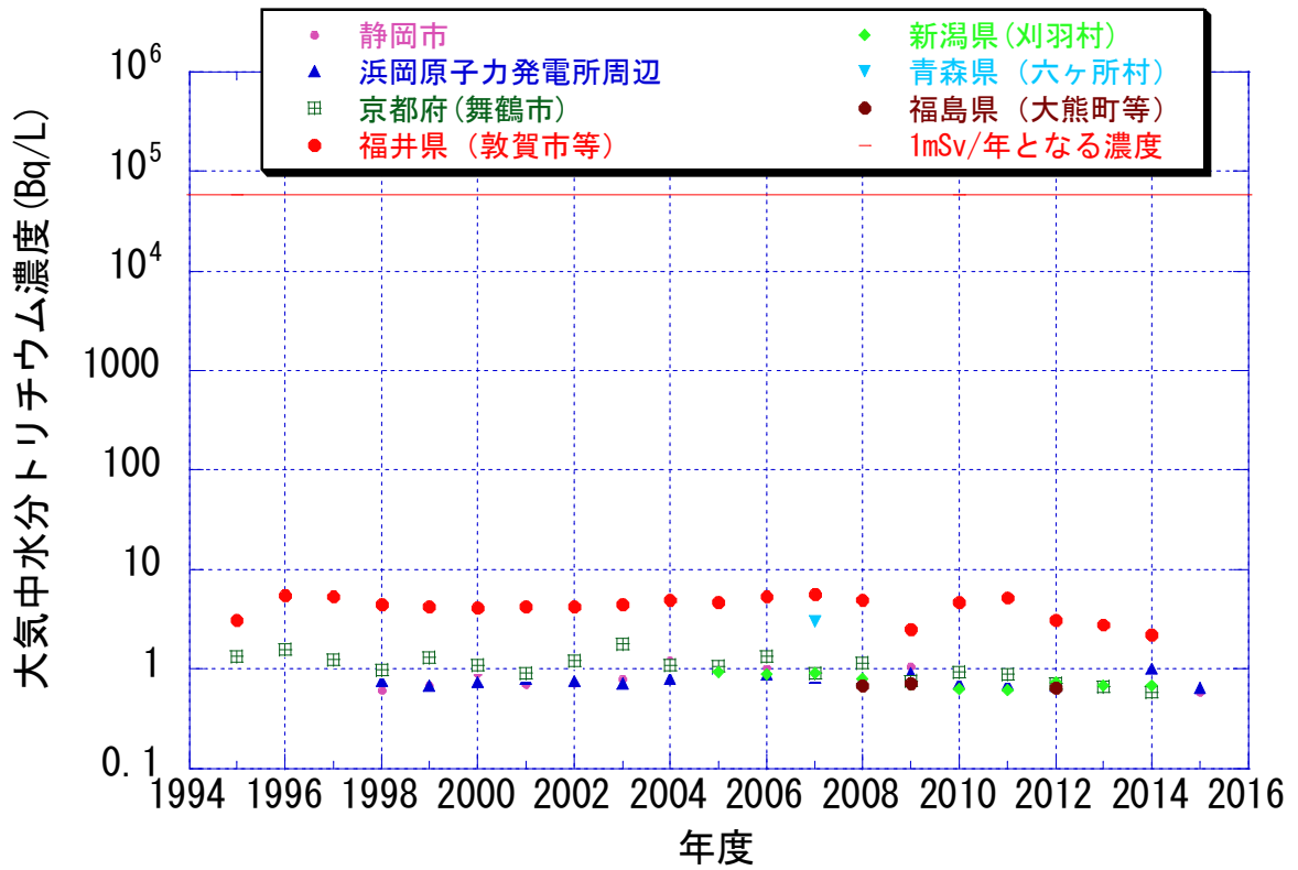
図9 大気中水分トリチウム濃度（年平均値）
