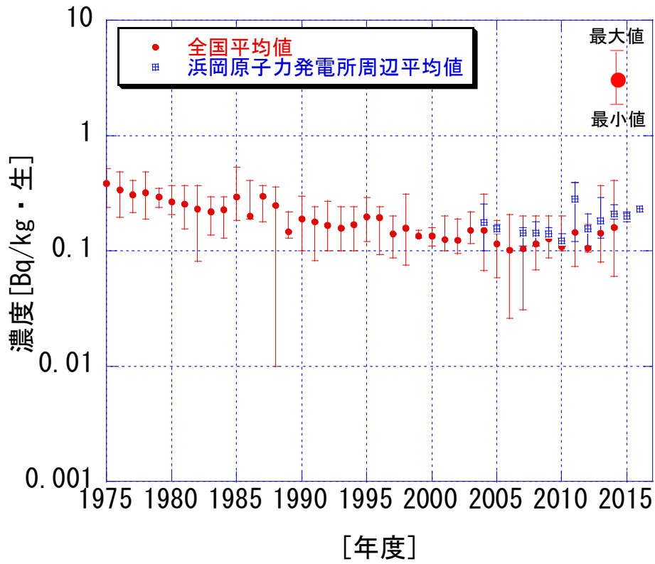
図7 あじ中の Cs-137 濃度
