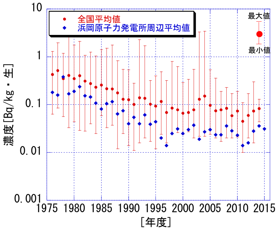
図8 大根中 Sr-90 濃度
