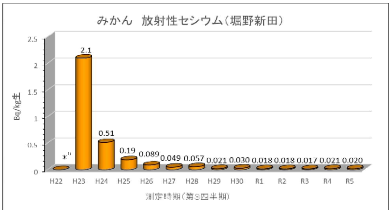
図2 みかん中の放射性セシウム濃度(Cs-134 と Cs-137 の合計量 2) )の経時的変化
