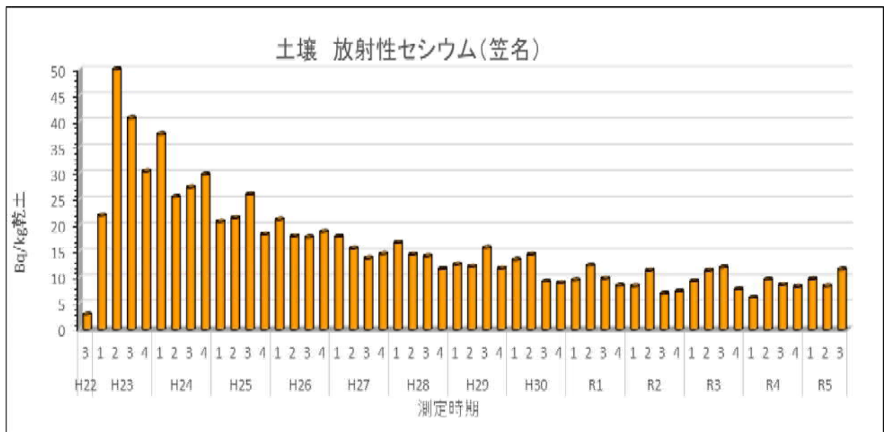
図1 土壌中の放射性セシウム濃度(Cs-134 と Cs-137 の合計量 1) )の経時的変化
