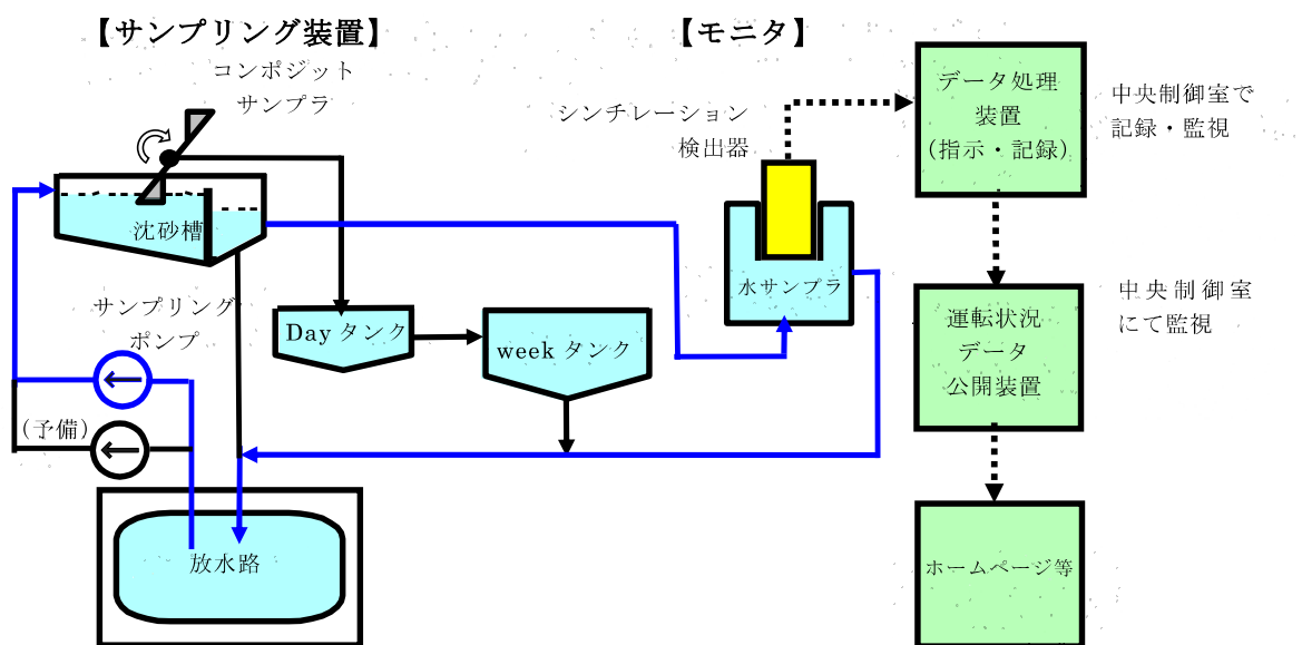
図2 放水口モニタに係る設備の概要
