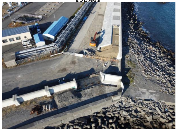
【施工中(胸壁)】
