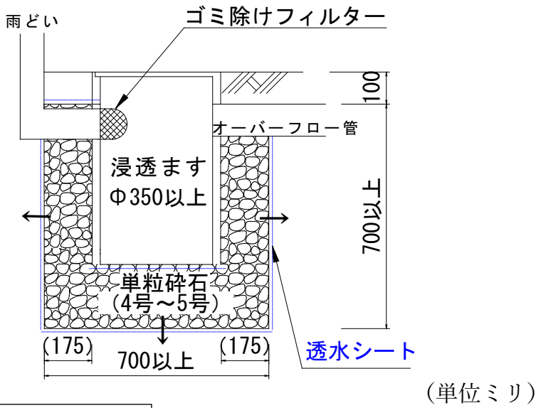
雨水貯留タンク
