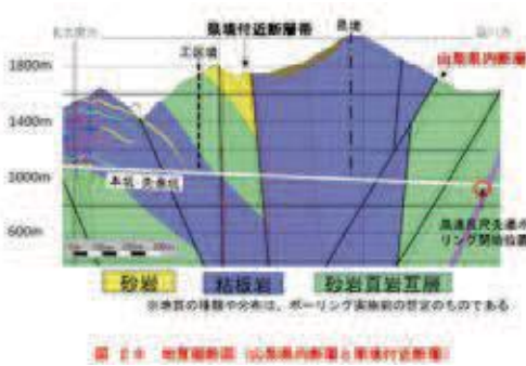
静岡工区の地質縦断面図 (静岡県HPから)
