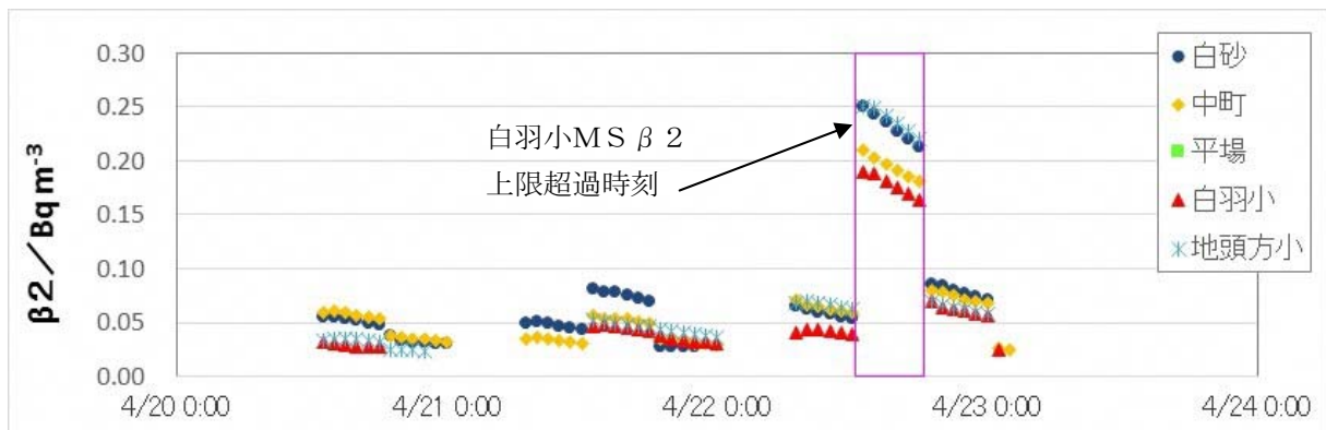
※LTD（検出限界未満）の測定結果は表示しない。 図3 各モニタリングステーションの浮遊塵中の全ベータ放射能（4月） （β2：集塵終了6時間後）
